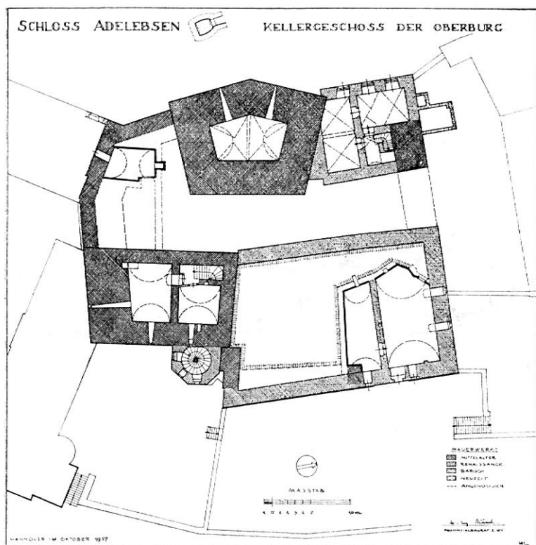
13. Schloß Adelebsen, Grundriß des Kellergeschosses der Oberburg (ehemalige Hauptburg).
