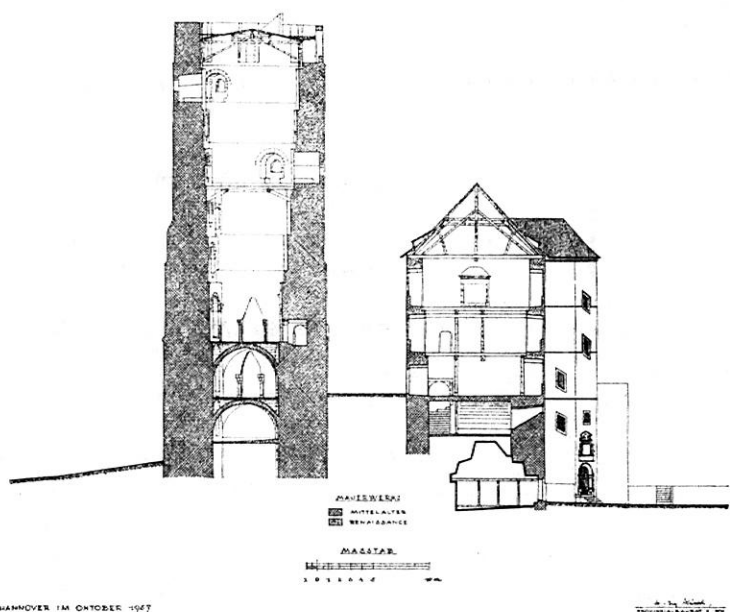
16. Schloß Adelebsen, Querschnitt durch die Oberburg (ehemalige Hauptburg) mit Wohnturm und Hinterhaus (heute als Mosthaus bezeichnet).
