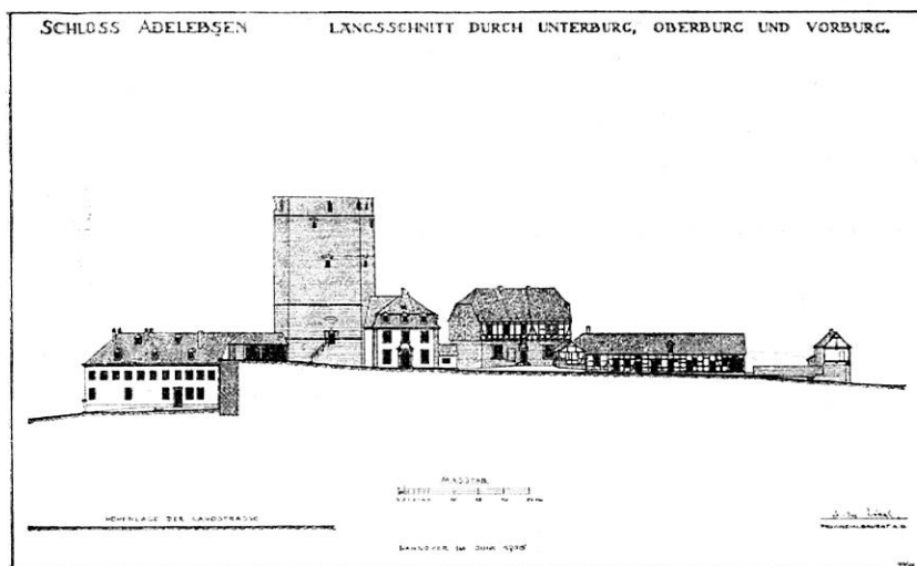
11. Schloß Adelebsen, Längsschnitt durch die Gesamtanlage.
